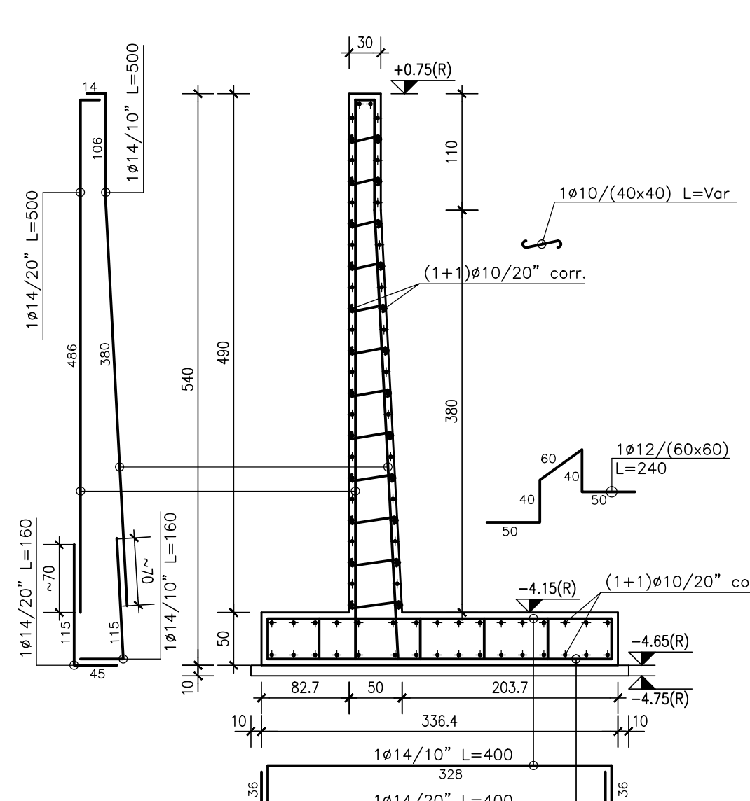
SEZIONE 2-2
