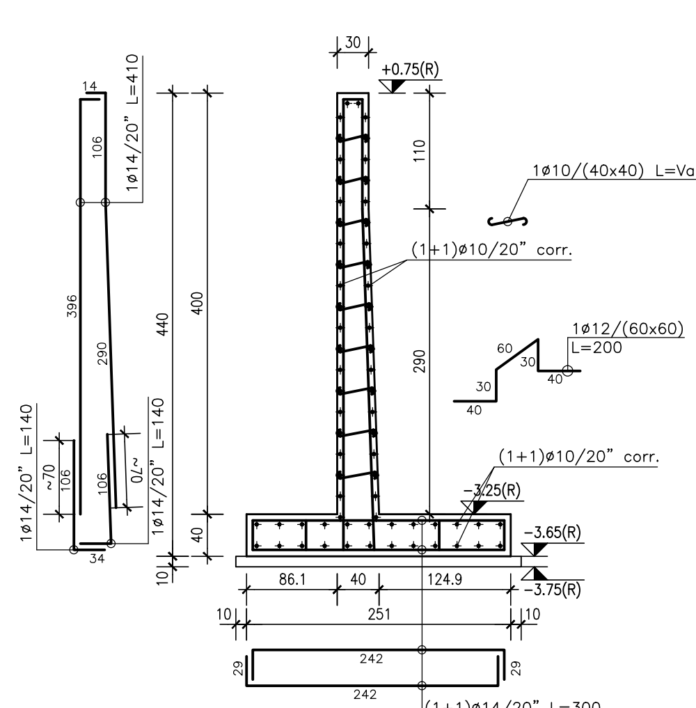
SEZIONE 3-3
