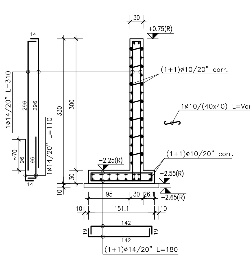
SEZIONE 4-4
