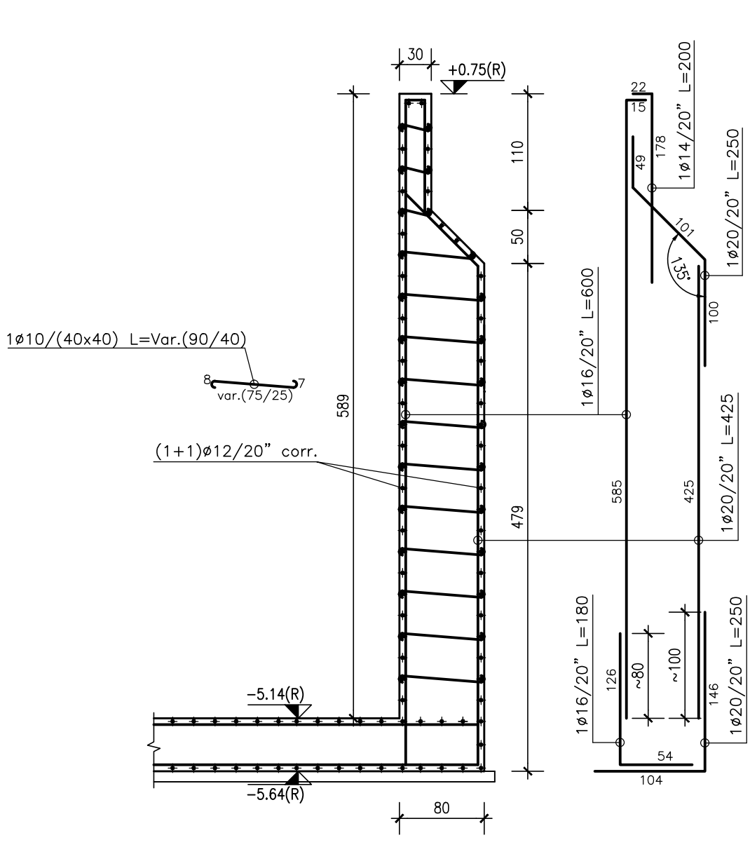
SEZIONE A-A
