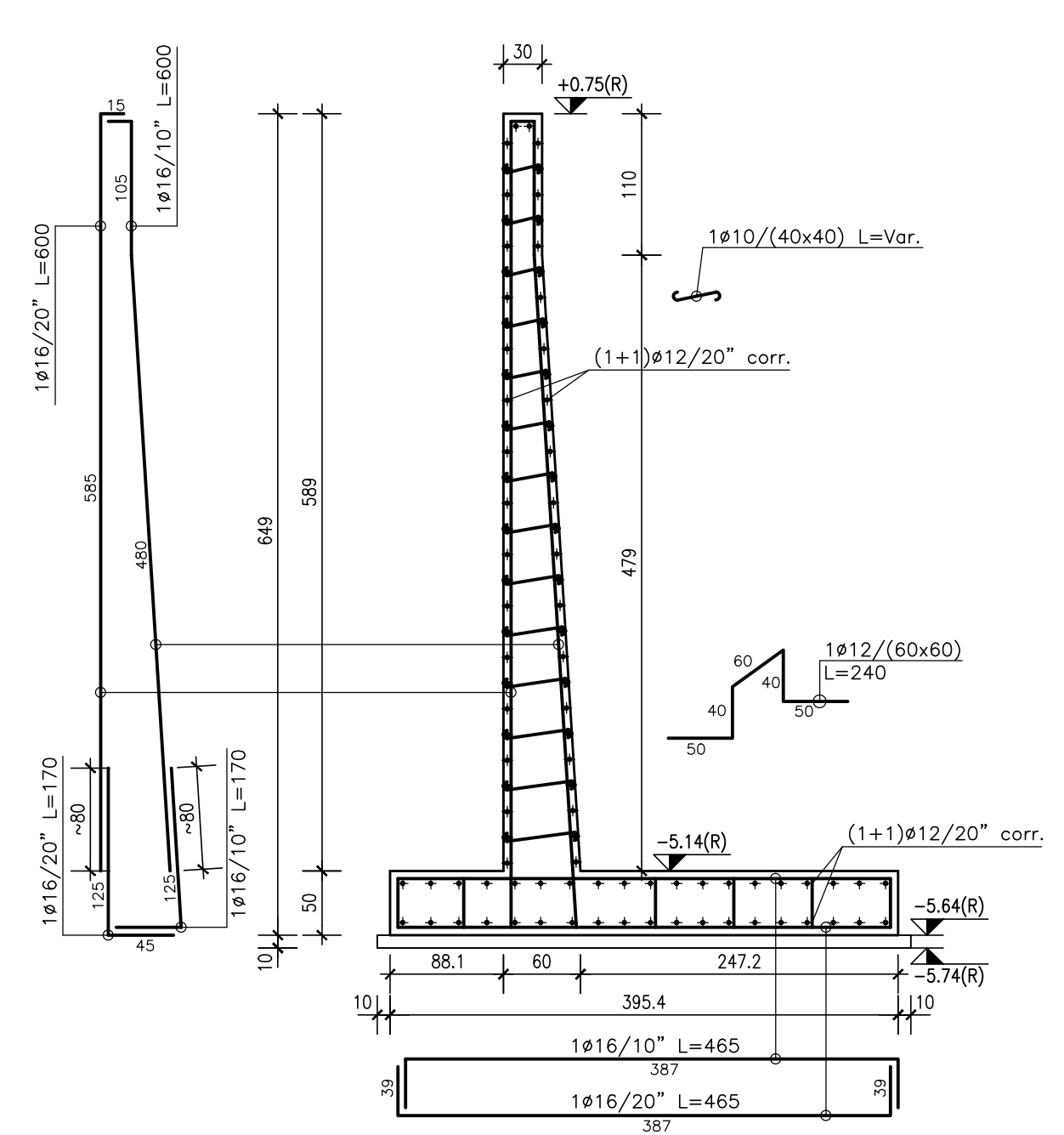
SEZIONE 1-1
